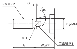
基準寸法表
