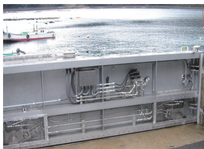
防潮堤
