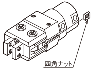
図1 締付トルク：0.4～0.6N・m
