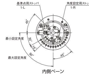
内側ベーン
