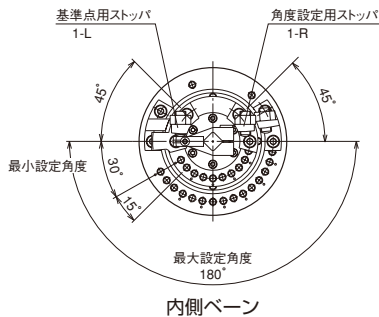
内側ベーン
